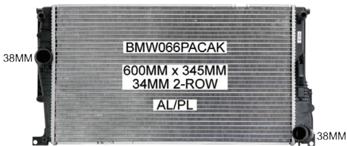
BMW F30/F31/F34 320i / 328i / 335i Auto. '12-
