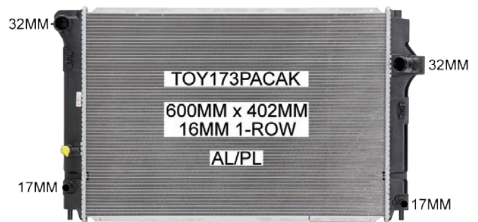
TOYOTA PRIUS C NHP10R Auto. '12-
